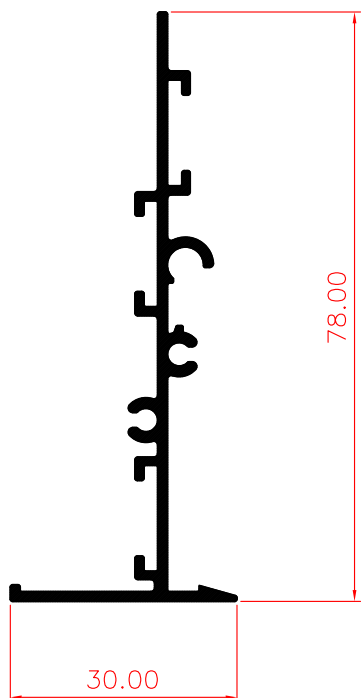
AVN-0025 | 0,575 kg/m
