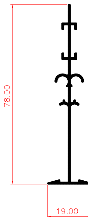
AVN-0024 | 0,396 kg/m
